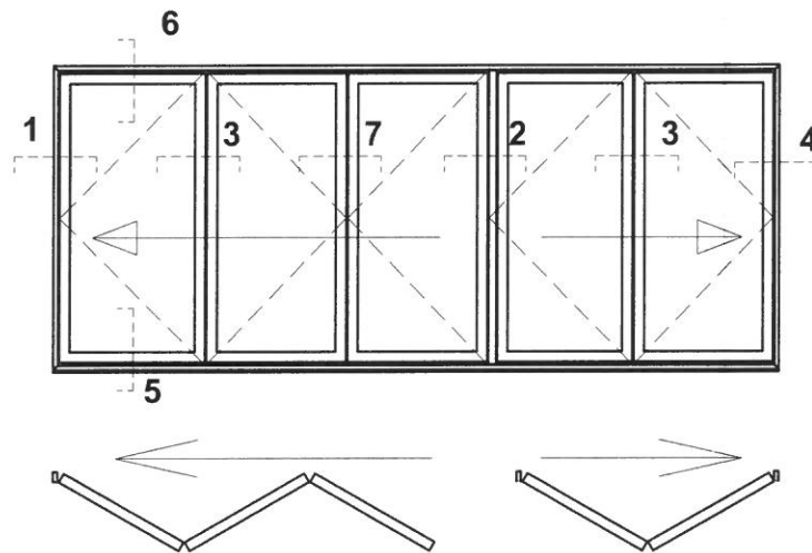
3/2 Split Door
